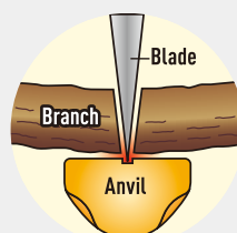
Anvil blade
