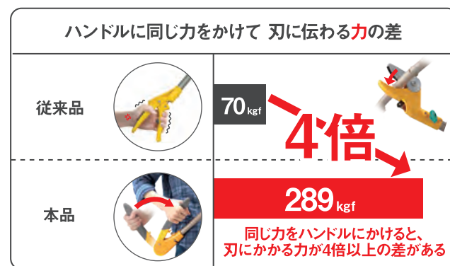
すご腕 3段式 プッシュカット アンビル刃 No.531
